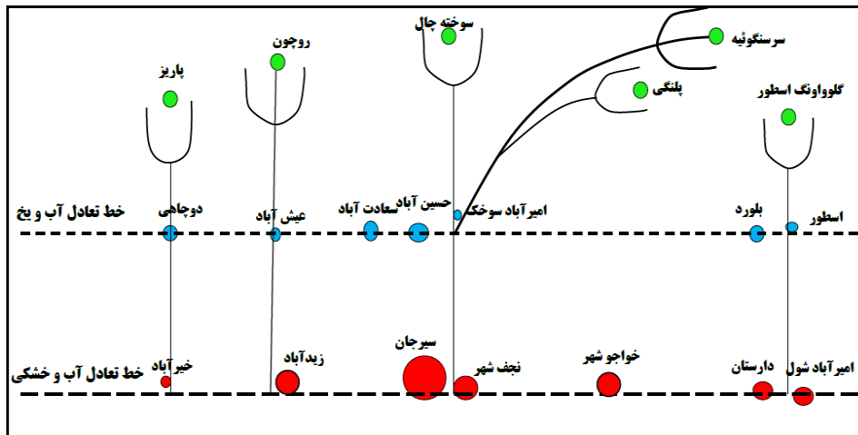
شکل ۷. چیدمان فضایی شبکه یخرودها و نسبت آنها با کانونهای جمعیتی
