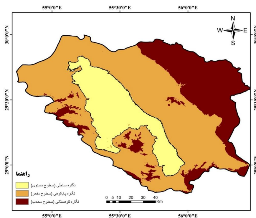
شکل ۳. تعیین حدود نگره‌های حوزه سیرجان
