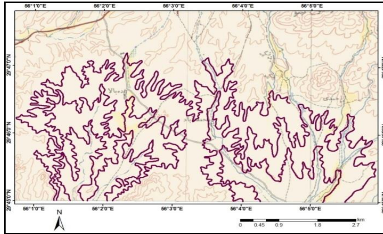
شکل ۵. آثار پهنه‌های یخی در نقشه‌های توپوگرافی حوزه سیرجان (نقشه توپوگرافی ۱/۵۰۰۰۰ اسمته (شماره 7249IV))
