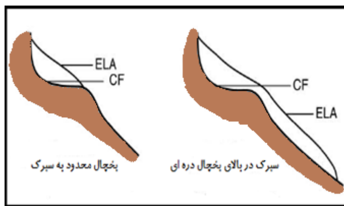
شکل ۲. روش ارتفاع کف سیرک (پورتر، ۲۰۰۱: ۱۰۶۹)
