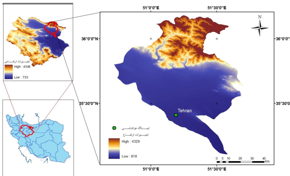
شکل ۱: موقعیت زیرحوضه و ایستگاه همدیدی انتخابی
