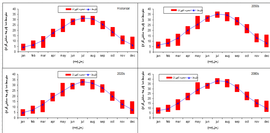
شکل ۱۱: محدوده تغییرات دمای متوسط دوره گذشته و تأثیرات تغییر اقلیم بر آن در دوره آتی مأخذ: یافته‌های تحقیق، ۱۳۹۱
