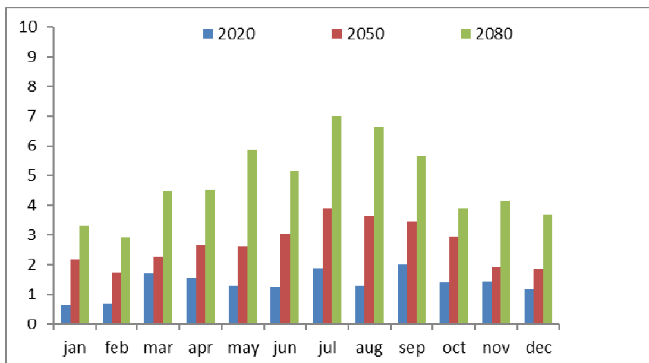
شکل ۶: سناریوی تغییر میزان دمای میانگین در صورت تغییر اقلیم طی سه دوره آینده
