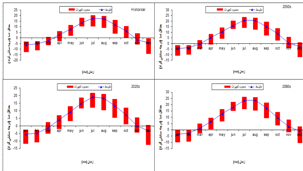
شکل ۹: محدوده تغییرات دمای حداقل دوره گذشته و تأثیرات تغییر اقلیم بر آن در دوره آتی
