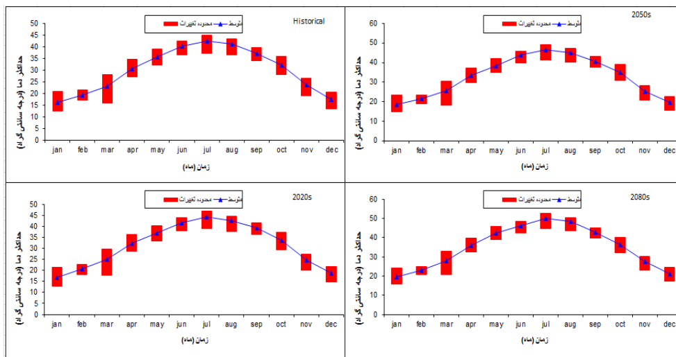
شکل ۱۰: محدوده تغییرات دمای حداکثر دوره گذشته و تأثیرات تغییر اقلیم بر آن در دوره آتی
