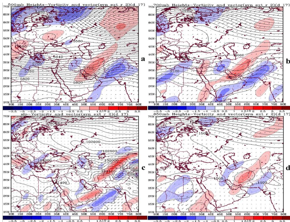
شکل ۴- ارتفاع ژئوپتانسیل (m)، تاوایی نسبی ( 10^{-5} )، جهت باد در سطح جوی ۵۰۰ (a)، ۷۰۰ (b)،
