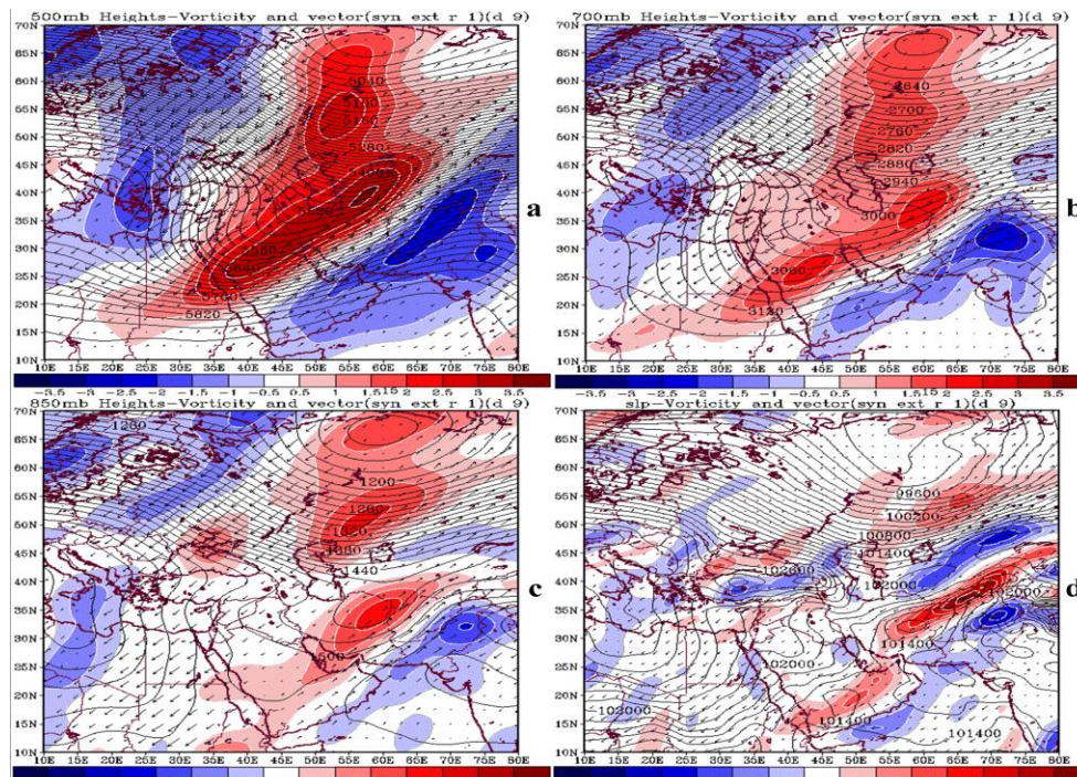
شکل ۲- ارتفاع ژئوپتانسیل (m)، تاوایی نسبی ( 10^{-5} ) و جهت باد در سطوح جوی ۵۰۰ (a)، ۷۰۰ (b)،
