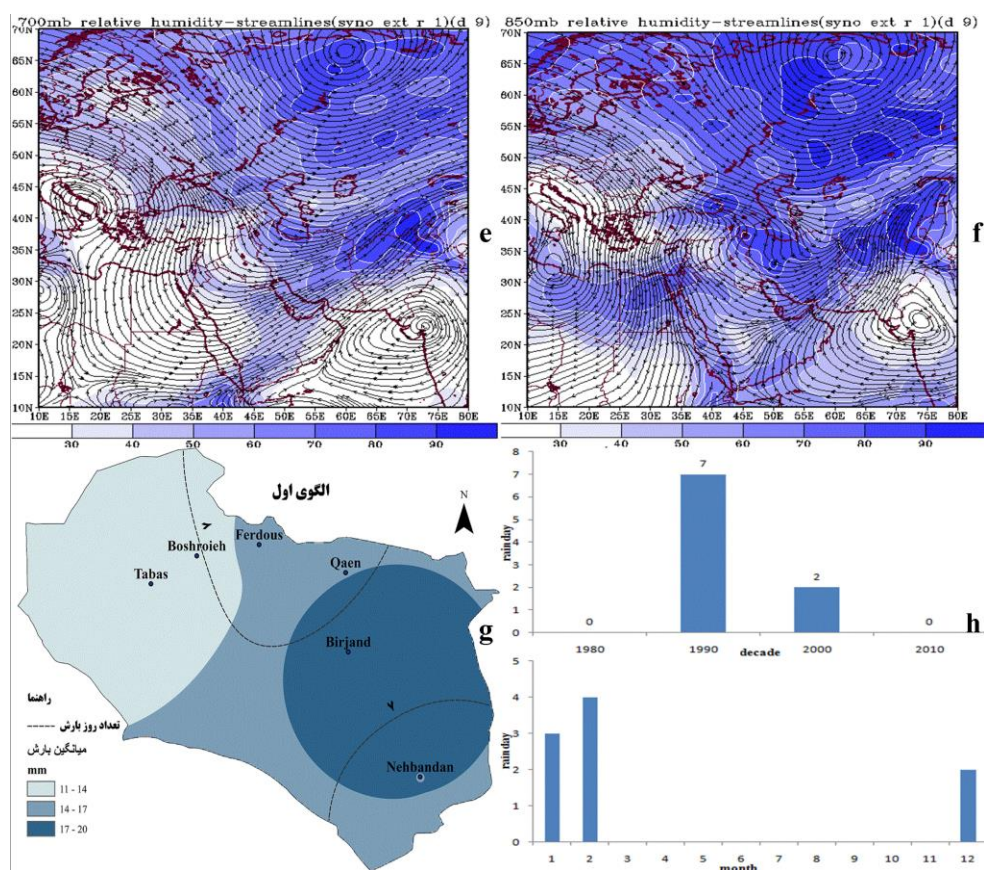
شکل ۳- خطوط جریان باد و رطوبت نسبی (%) سطوح جوی ۷۰۰ (e)، ۸۵۰ (f) میلی بار و توزیع
