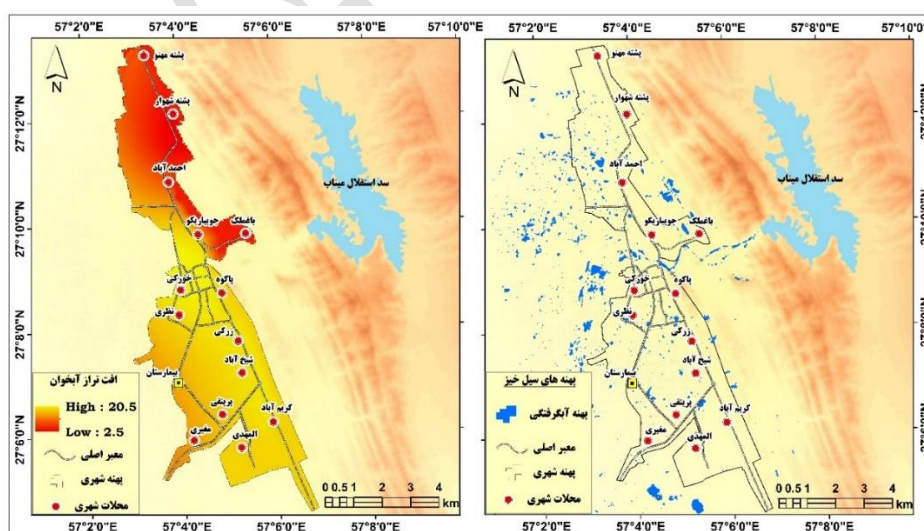
شکل ۳. وضعیت افت تراز آبخوان میناب و پهنه‌های آب‌گرفتگی (تصویر ماهواره‌ای ستینل ۲)
